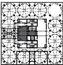
Erdgeschoss
